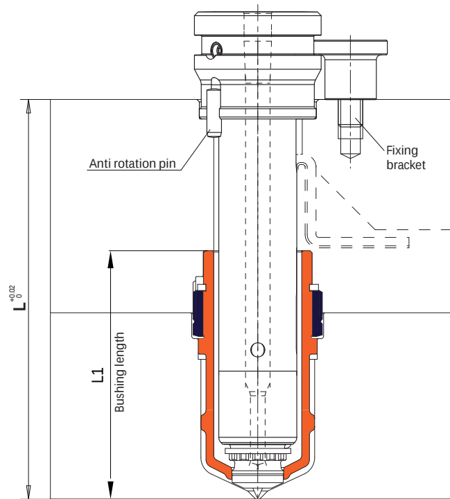
sez B-B
