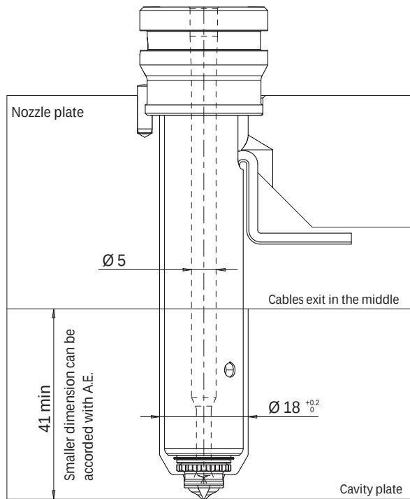
sez A-A
