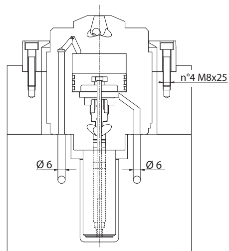
SEZ. C-C
